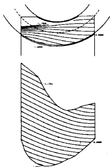
Computerbestimmte Berührungsfläche und -linien zur Überprüfung der Konstruktion jedes einzelnen Schneckenradsatzes.
