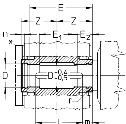
(a) Albero lento cavo con cava linguetta
