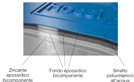
Strati di verniciatura Classe C5-M
