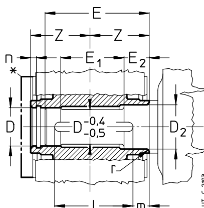
(b) Albero lento cavo differenziato con cava linguetta
