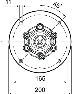
F320 Ø 200
